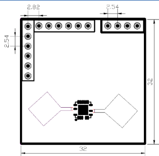
图 6 整体尺寸(32mm*32mm*2.5mm)
