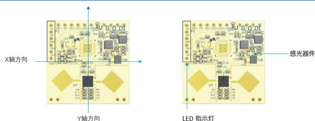
图 5 感知方向和光感器件
